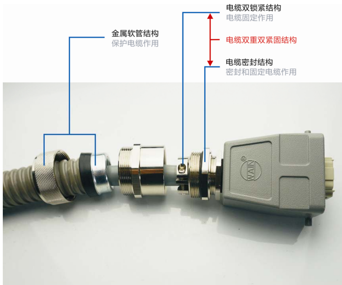
装配后的整体结构示意图 整体的防护等级是IP65
