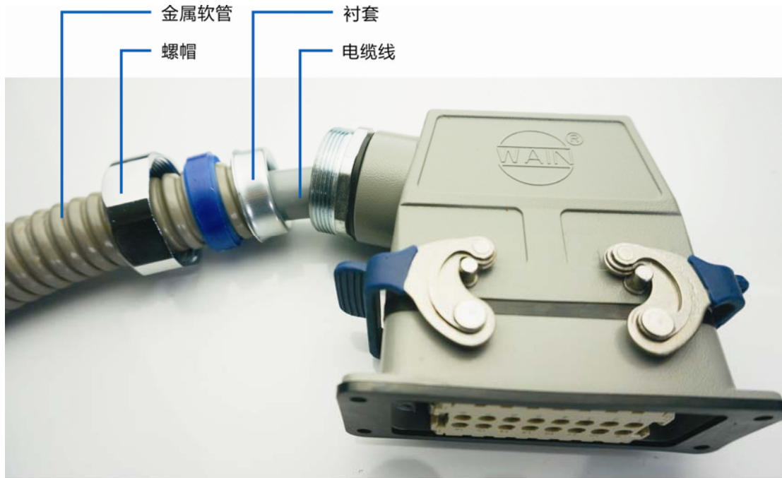
装配后的整体结构示意图
